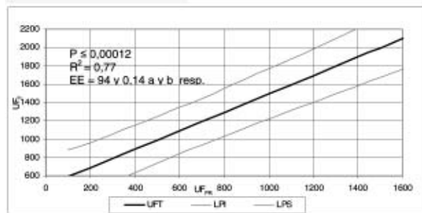
Figura 2. Relación entre las UFUM_{FR} observadas el 20-07 (201 DJ) y las UFUM_{TO} con sus respectivos límites de predicción 90% confianza Luján de Cuyo.
