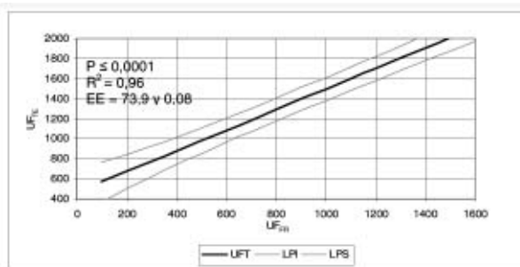
Figura 6. Relación entre las UF_{FR} observadas el 01-08 (213 DJ) y las UF_{TE} y sus límites de límites de predicción, 90% confianza. Tupungato. Figure 6. Relationship CU at the reference date 01-08 (213 Julian day) and total CU estimated and its predictions limits 90% of confidence Tupungato.
