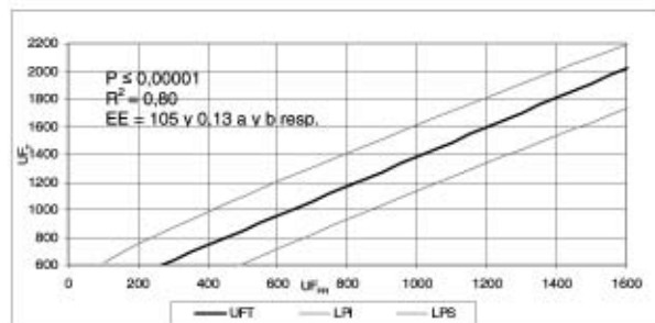
Figura 3. Relación entre las UFUM_{FR} observadas el 01-08 (213 DJ) y las UFUM_{TE} y sus límites de predicción 90% confianza, Luján de Cuyo.
