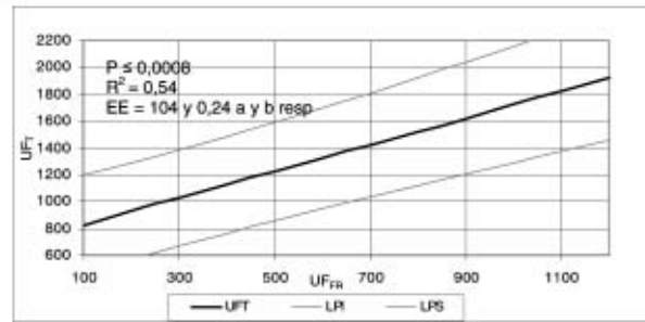
Figura 1. Relación entre las UFUM_{FR} observadas el 01-07 (182 DJ) y las UFUM_{TO} y sus límites de predicción 90% confianza Luján de Cuyo.
