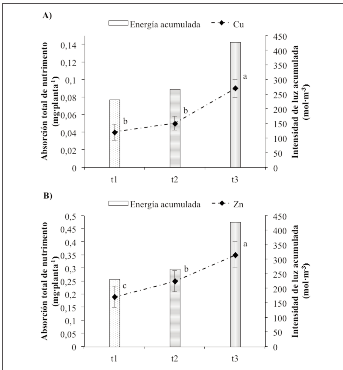
Figura 2. Absorción total de nutrimentos por planta, A) Cu y B) Zn, en el cultivo de lechuga romana tipo baby en base a peso seco (raíz + hojas) a los 21 días después de trasplante bajo tres tratamientos de intensidad de luz ( t1 = 127,49 \mu\text{mol}\cdot\text{m}^{-2}\cdot\text{s}^{-1} ; t2 = 147,32 \mu\text{mol}\cdot\text{m}^{-2}\cdot\text{s}^{-1} y t3 = 235,69 \mu\text{mol}\cdot\text{m}^{-2}\cdot\text{s}^{-1} ) cultivada en un Sistema Plant Factory ( \bar{x} \pm \text{DE} , n = 14 ).
